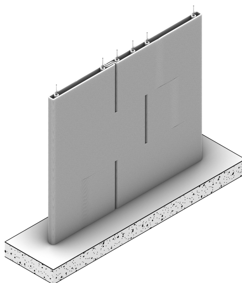
4_ Compleción del muro y anclaje superior
