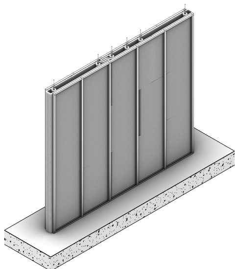
5_ Montaje de la subestructura metálica para placa de yeso
