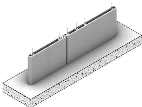
3_ Colocación de las armaduras de conexión para la hilada superior
